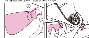
QSV-1サンバイザーの取り付け方 Installing the QSV-1 Sun Shield / Visor
