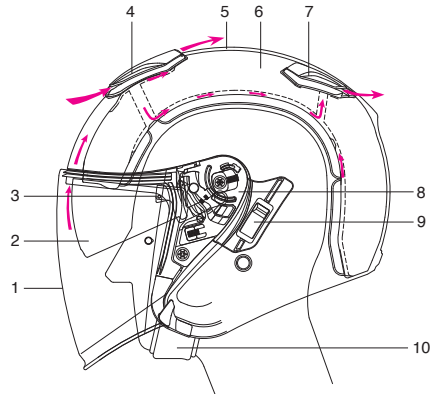
Visiirin huurtumista estävä ilmanvaihtojärjestelmä Visirventilationssystem mot kondensering
