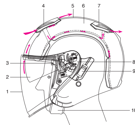
Σύστημα εξαερισμού κατά της θάμβωσης της ζελατίνας System wentylacji zapobiegający zaporowaniu osłony
