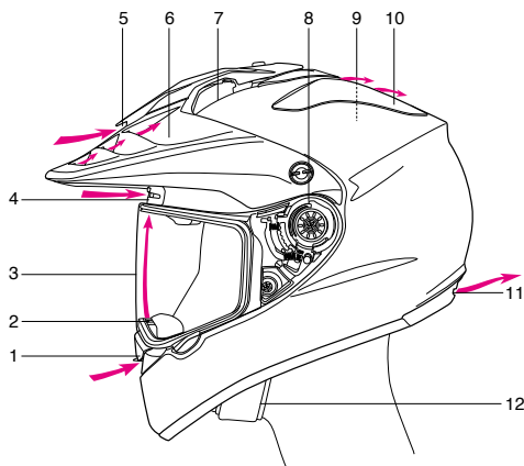
Vorderer Ventilationseinlass Preso di ventilazione frontale
