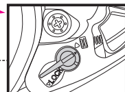
Μοχλός κλειδώματος σκανδάλης ζελατίνας Δζωιγνια βλοκωвания οσλόνης z cynglem
