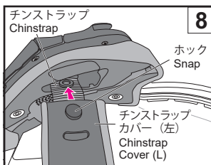
チンストラップカバー (左) Chinstrap Cover (L)
