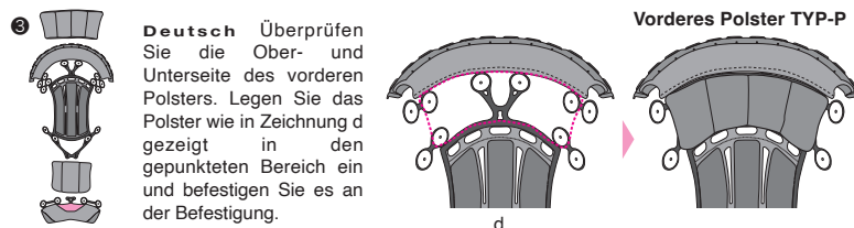
Vorderes Polster TYP-P
