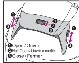
Upper Air Intake Entrée d'air supérieure
